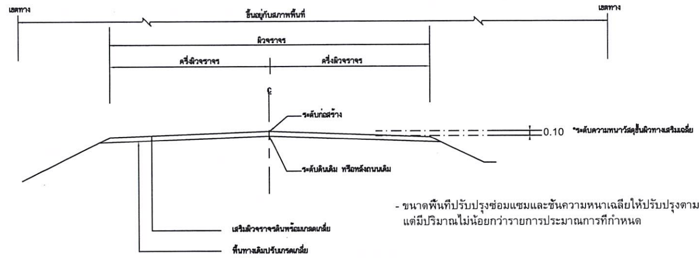
รูปตัดโครงสร้างทาง NO SCALE
