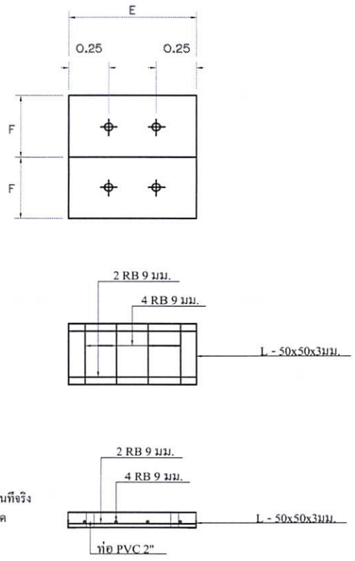
แบบขยายฝาบ่อพัก
