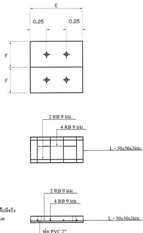
แบบขยายฝาบ่อพัก
