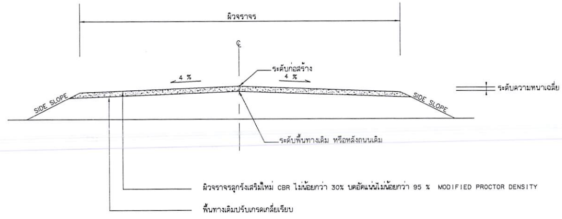
รูปตัดดีโครงสร้างทาง NO SCALE
