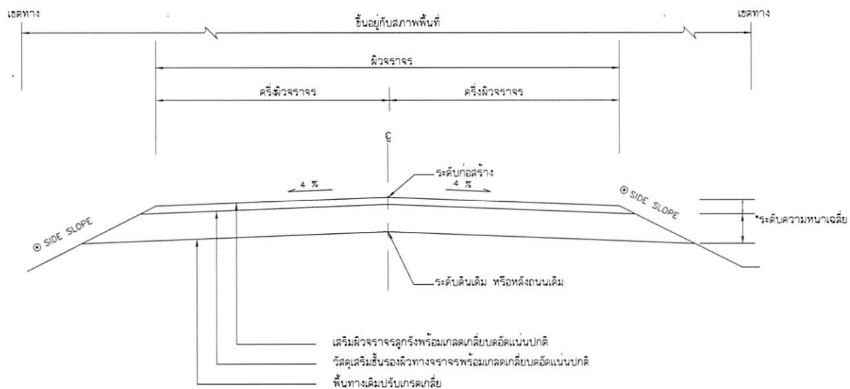
รูปตัดโค้งโครงสร้างทาง
