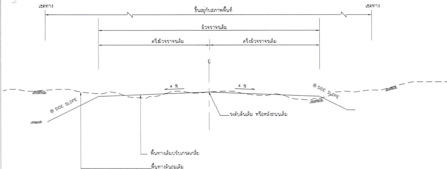
รูปตัดโค้งโครงสร้างทางเดิม
