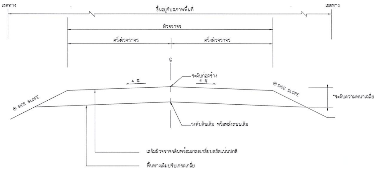
รูปตัดดีโครงสร้างทาง NO SCALE
