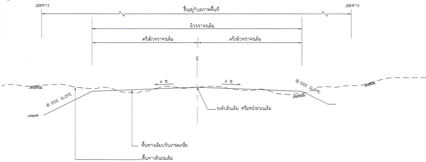
รูปตัดดีโครงสร้างทางเดิม NO SCALE
