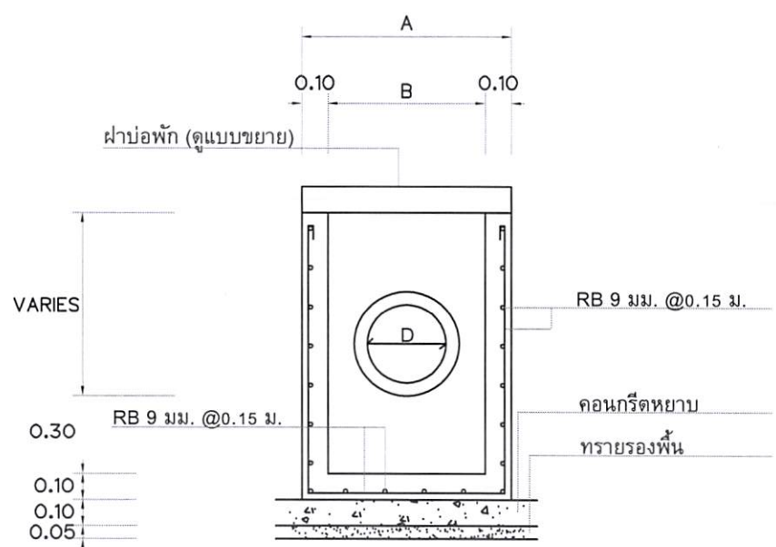
รูปตัดบ่อพัก คสล.
