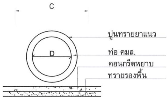
รูปตัดบ่อพัก คสล.
