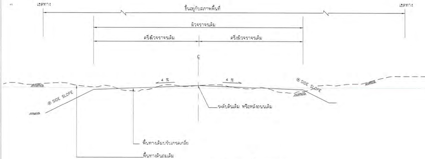
รูปตัดโครงสร้างทางเดิม
