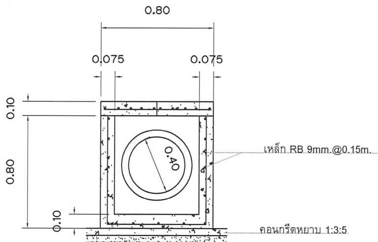
รูปตัดบ่อพัก
