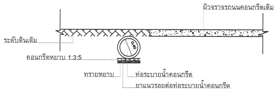
รูปตัดแนววางท่อ
