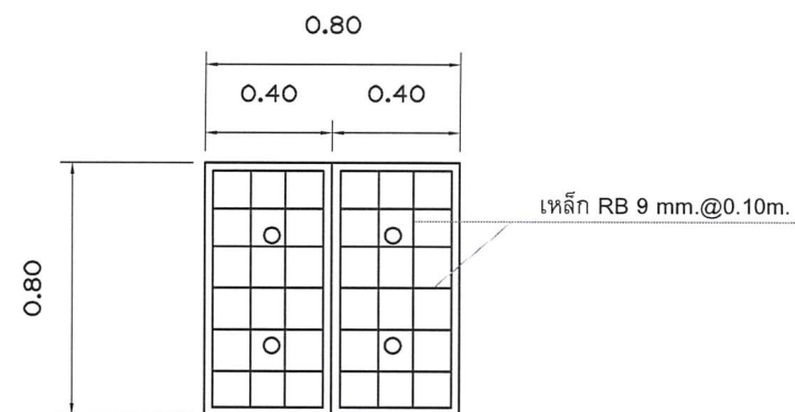
แบบแปลน
