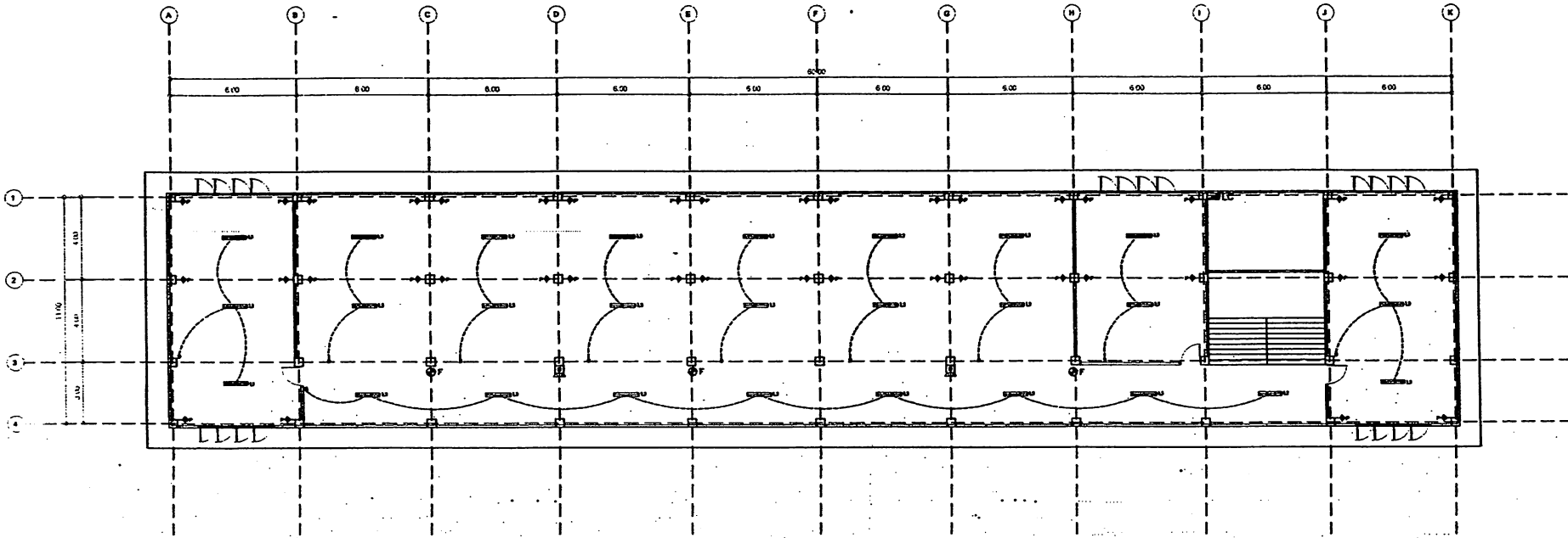
แปลนไฟฟ้าชั้น 1
