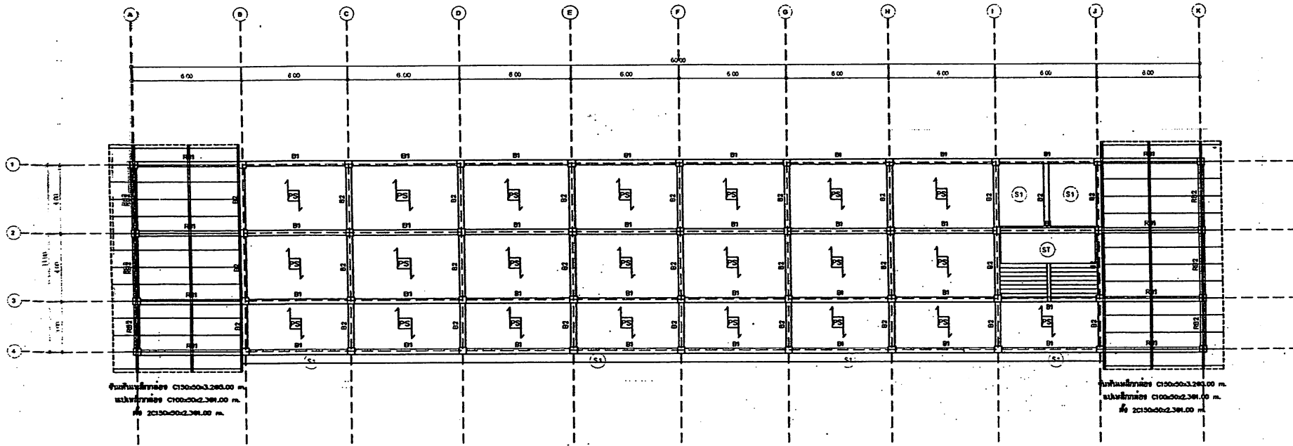
แปลนโครงสร้างชั้น 2
