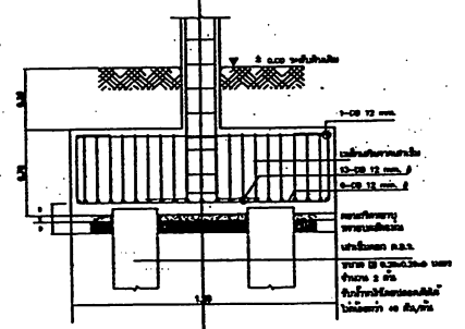
F1 Section 1:25
