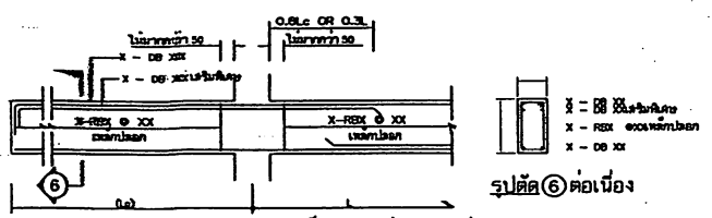
แบบมาตรฐานแสดงการเสริมเหล็กในคานยื่น แบบที่ (1)
