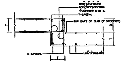
แบบมาตรฐานแสดงการเสริมเหล็กในคานยื่น แบบที่ (1)
