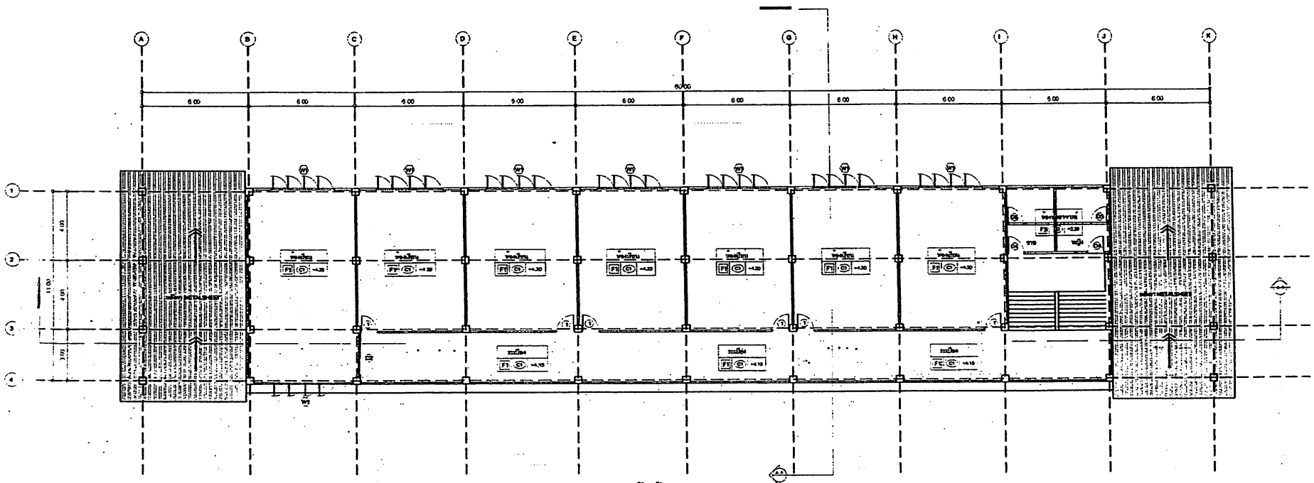
แปลนพื้นชั้น 2
