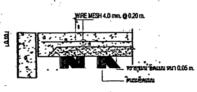
แบบขยายพื้น GS มาตราส่วน 1 : 25
