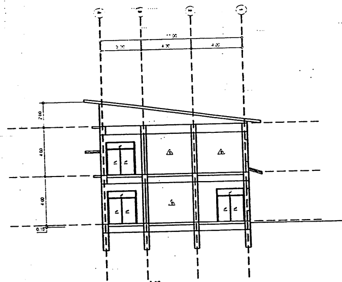
รูปตัด B-B
