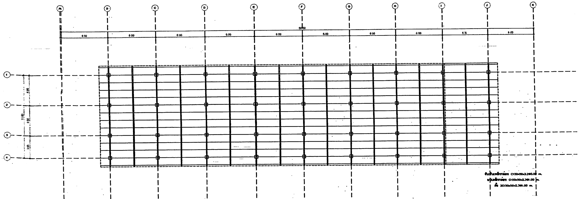
แปลนโครงสร้างหลังคาเหล็ก
