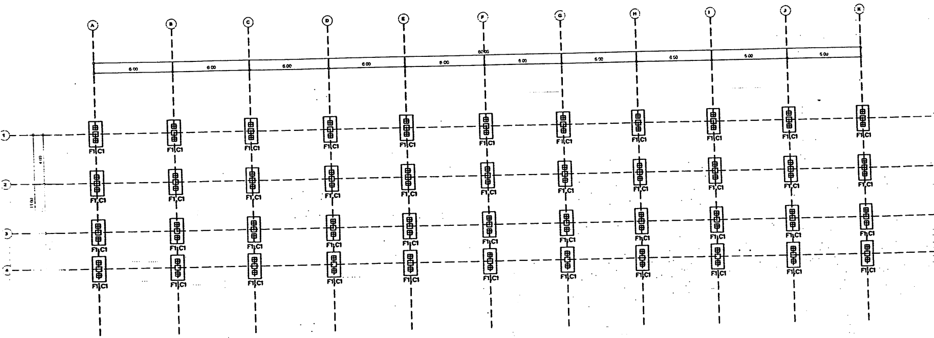
แปลนฐานรากเสาเข็ม
