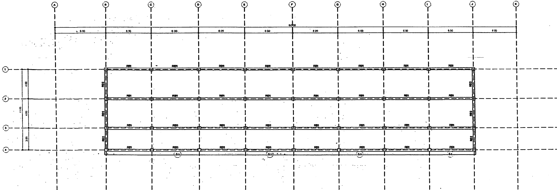
แปลนโครงสร้างหลังคา คสล.
