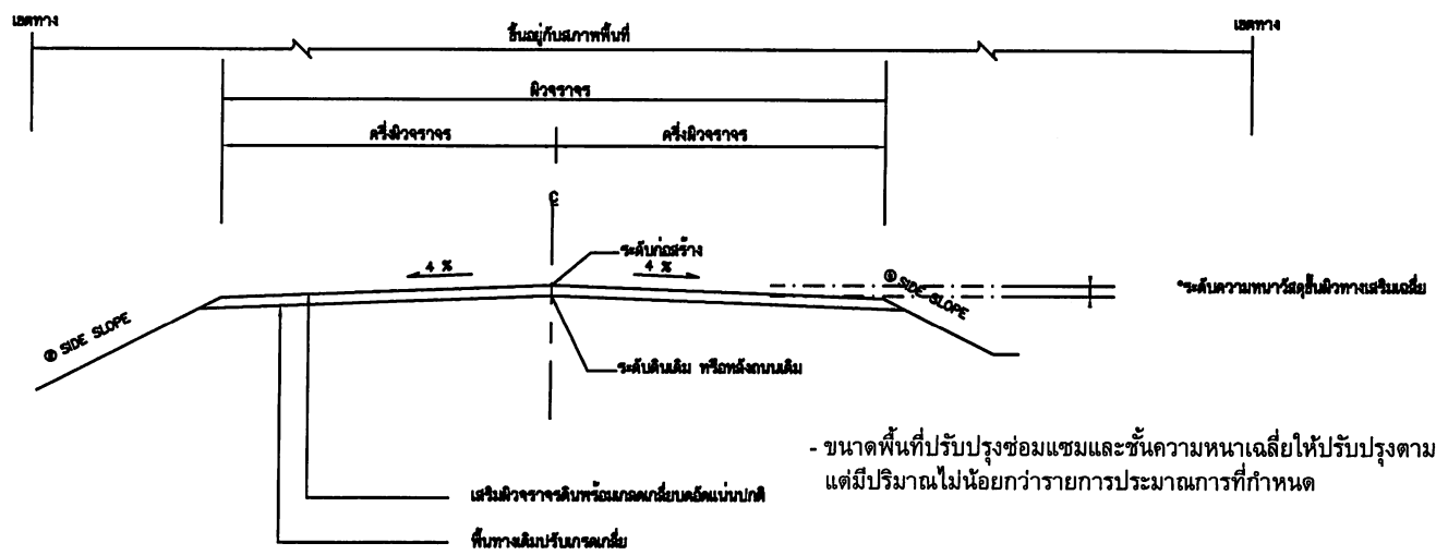
รูปตัดโครงสร้างทาง NO SCALE
