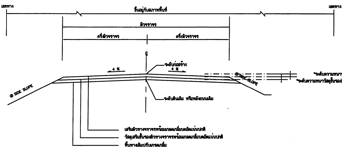
รูปตัดโครงสร้างทาง NO SCALE
